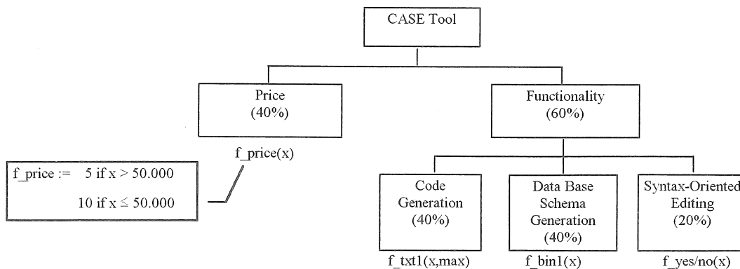
Figure 4 - An EM Model
